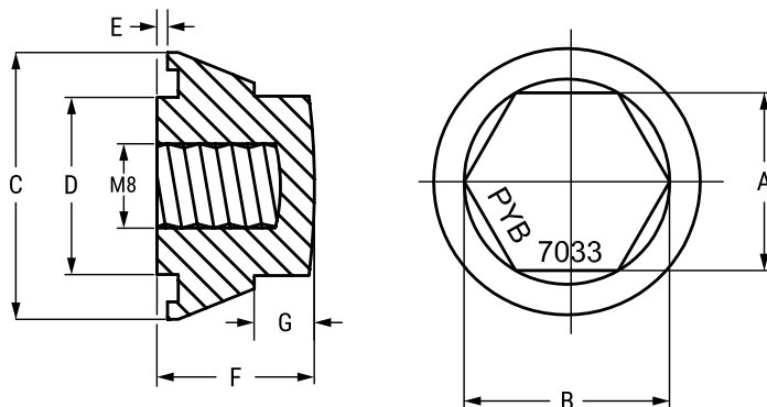
M8 Nut
