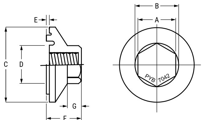
M12 Nut
