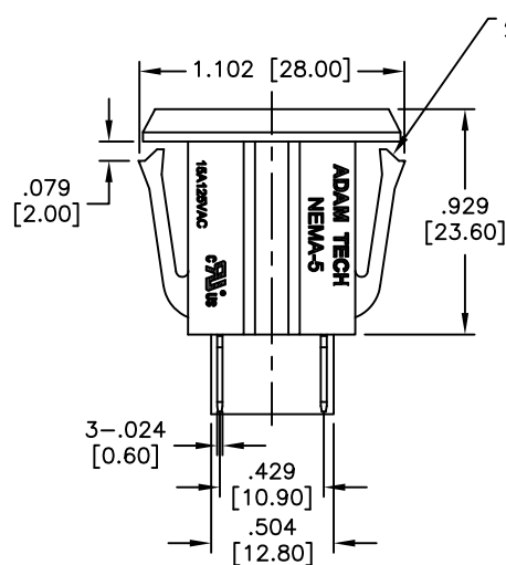
SECTION A-A
